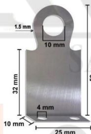
KRM-K-PDE-R-DL52
