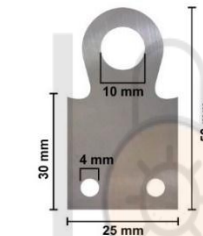
KRM-K-PDE-F-L50
